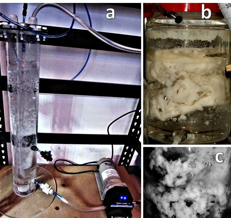
Figura 3. Sistemas de tratamiento de efluentes gaseosos: a) módulo de oxidación controlada de H_2S de un sistema de desulfuración en dos etapas; b) sistema multifásico de segunda generación para la eliminación de VOC; y c) detalles de aceite de silicón colonizado con bacterias hidrofóbicas degradadoras de hexano.
