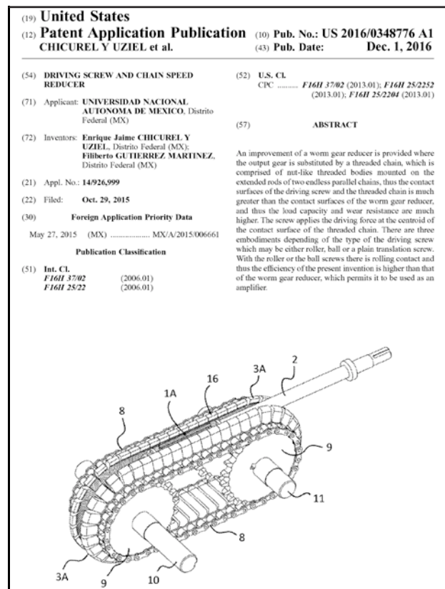
Figura 2. Solicitud de patente estadounidense de la segunda versión del reductor de velocidad
