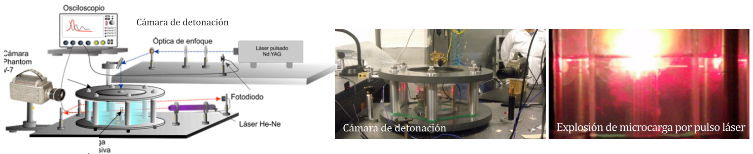
Figura 5. Cámara de detonación para el estudio de microcargas explosivas detonadas por pulso láser
