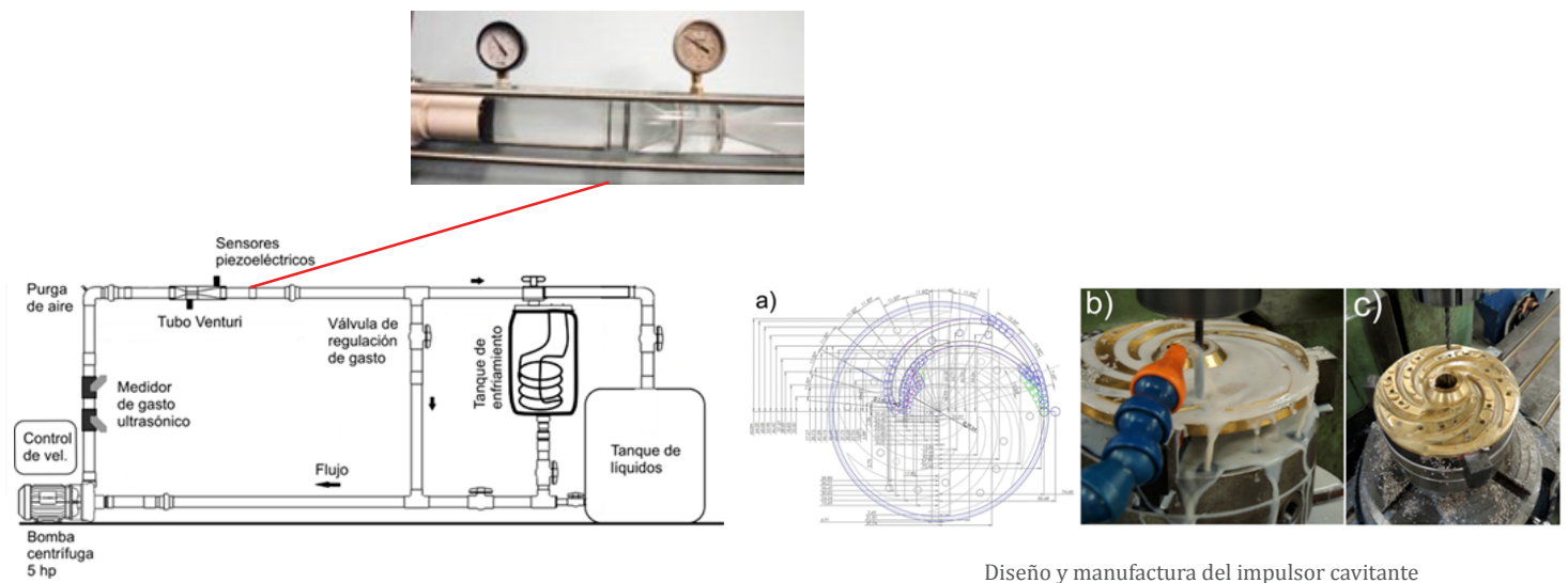
Diseño y manufactura del impulsor cavitante
