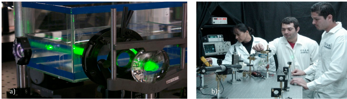
Figura 1. a) Cavitación por pulso láser, b) Sonoluminiscencia de una sola burbuja
