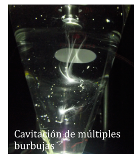
Figura 2. Aparato para el estudio de muchas burbujas usando campos acústicos en reactor cónico
