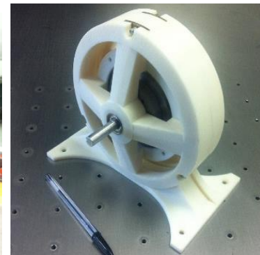
Figura 5. Reductor de velocidad ligero de engranes magnéticos del IUNAM
