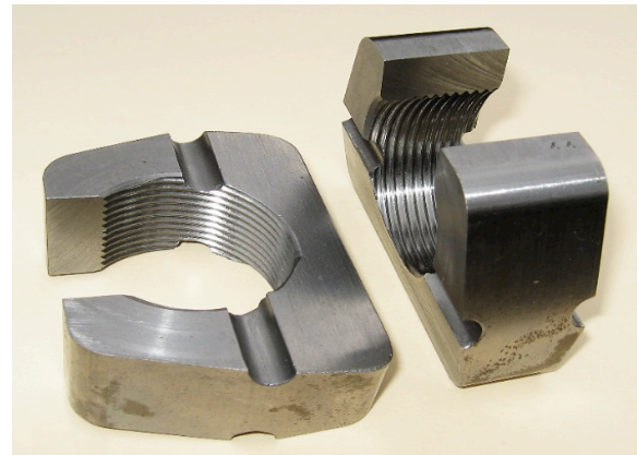
Figura 7. Cuerpos roscados. Las depresiones semicilíndricas son los alojamientos de los pernos extendidos de dos cadenas de rodillos; sus ejes están en el plano horizontal que contiene al centroide de la superficie cilíndrica, interna roscada
