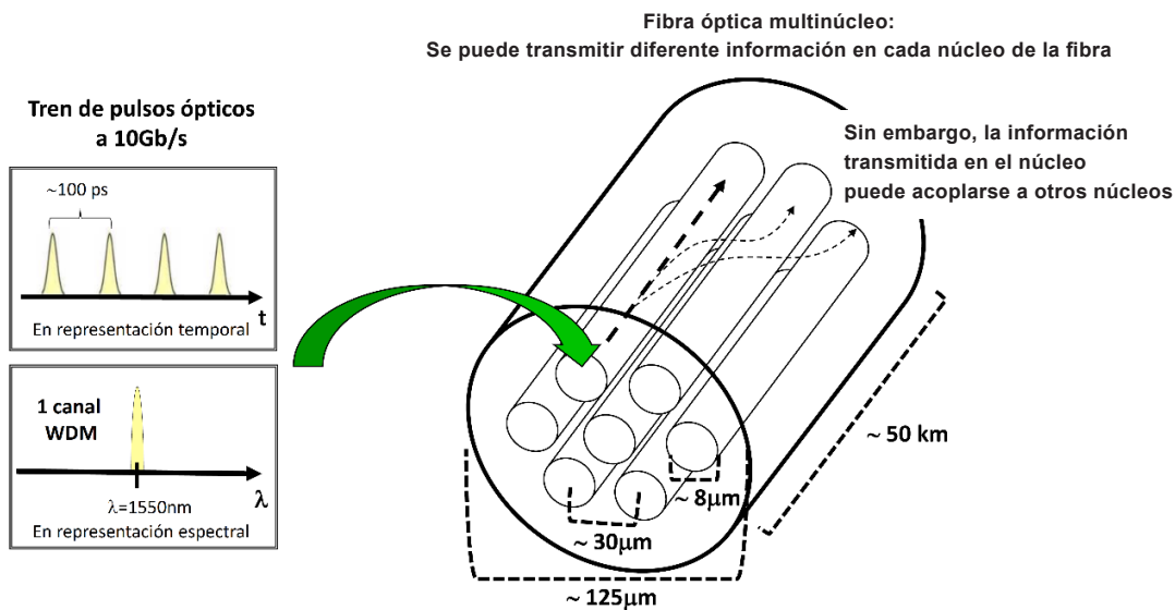
Figura 1. Transmisión de señales en fibras ópticas multinúcleo
